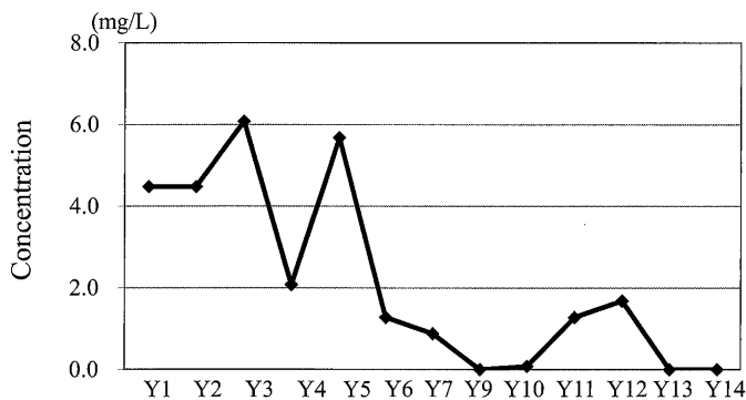
図5 大和川におけるフミン酸の濃度の変化
